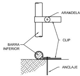
DETALLE ANCLAJES
