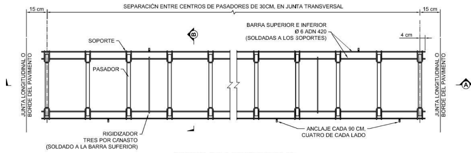
CANASTO DE PASADORES VISTA EN PLANTA
