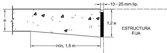
TIPO F-2 JUNTA DE AISLACIÓN CON SOBRE-ESPESOR
