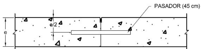
TIPO B JUNTA TRANSVERSAL DE CONSTRUCCIÓN
