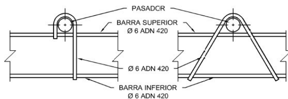
SOPORTE TIPO "J"
