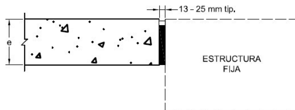
TIPO F-1 JUNTA DE AISLACIÓN
