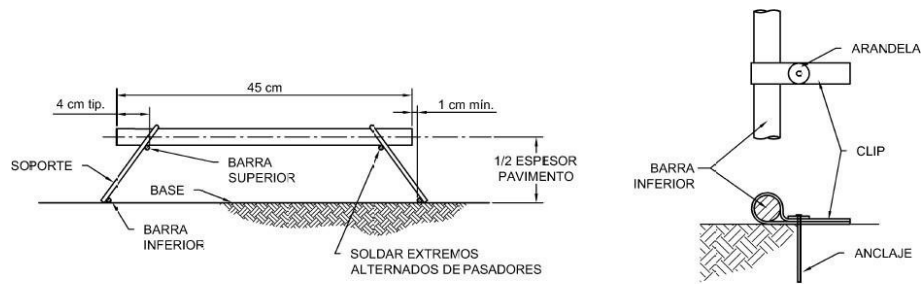
CORTE (B)
