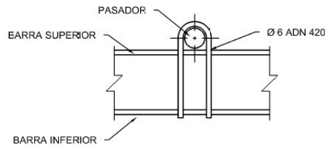
SOPORTE TIPO "U"
