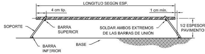
CORTE (B)
